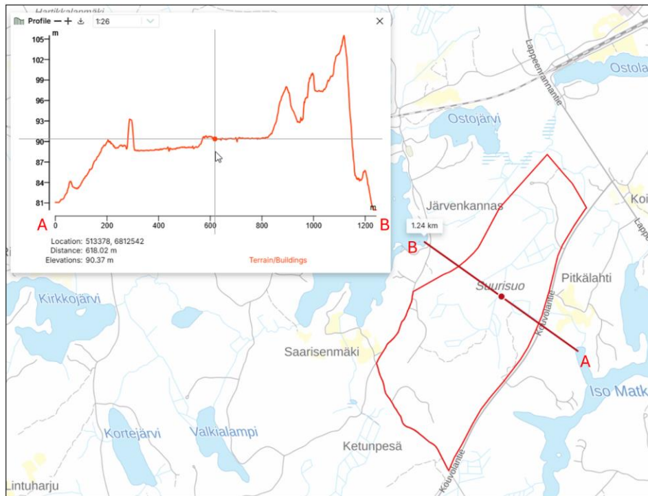
Kuva 13. Alueen korkeusprofiili kaakkois-luoteissuunnassa (Scalgolive, 2025).
