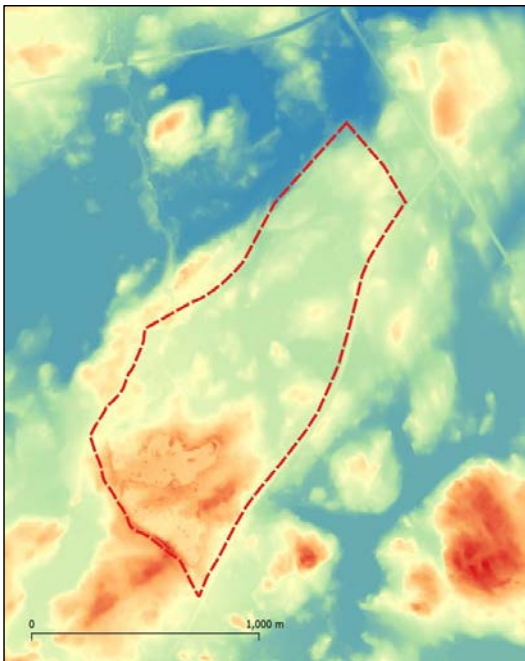
Kuva 11 Suunnittelualueen korkeussuhteet. (Maanmittauslaitos)
