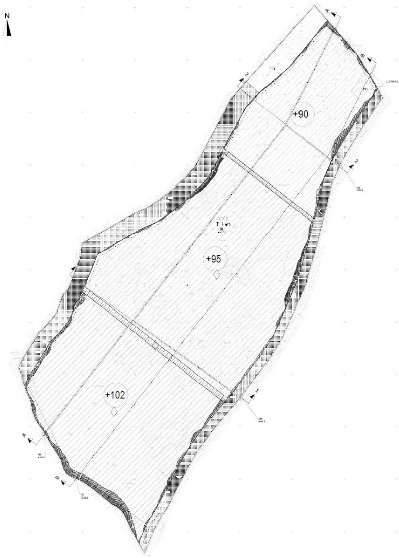
Kuva 45. Yleistasaus porrastettu malli +90 m, +95 m ja +102 m.
