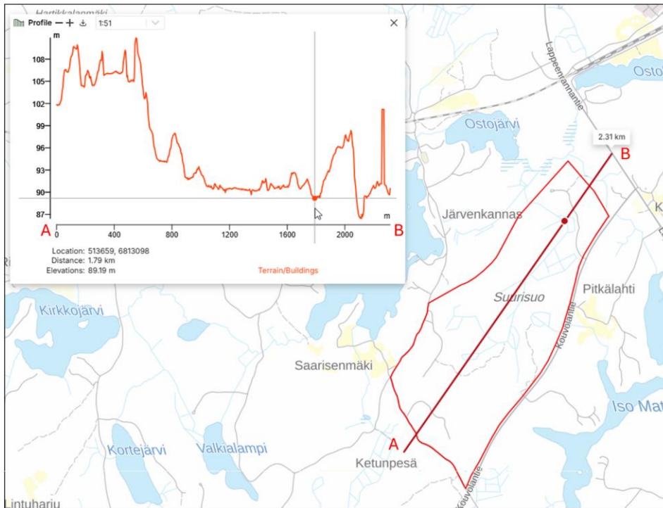
Kuva 12. Alueen korkeusprofili lounais-koillissuunnassa (Scalgotlive, 2025).
