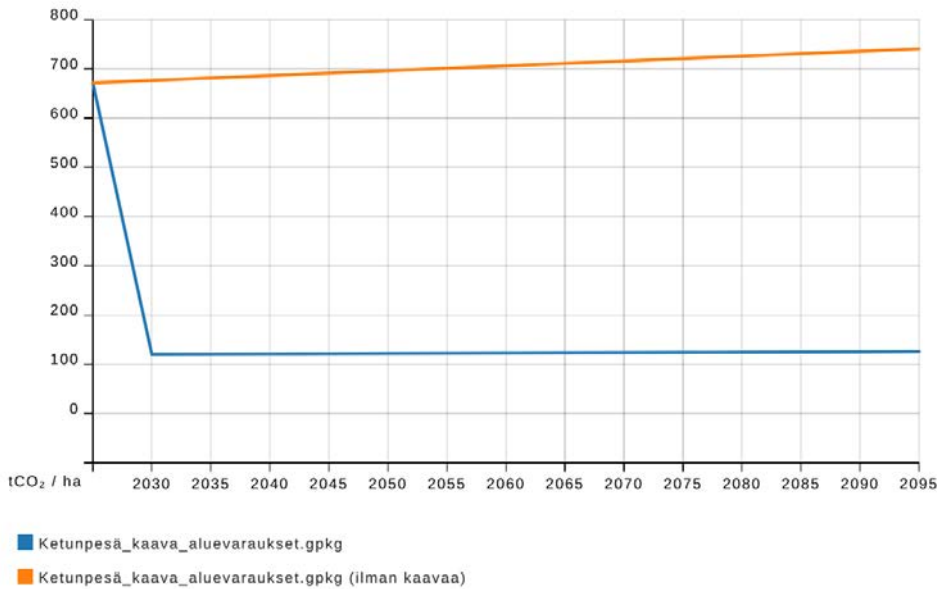
Kuva 51. Hiilivaraston muutos kaava-alueella yhteensä. (hiilikartta.avoin.org)
